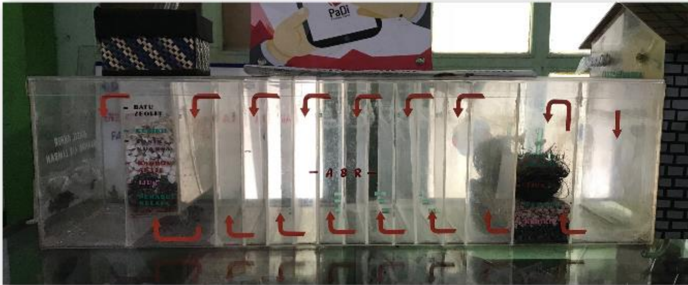
Gambar 4 Maket Pandora L (Pendaur Ulang Air Limbah) (Dok: Penulis)
